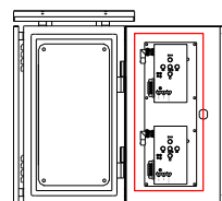
扉裏側「MDR-264A」2台の取付イメージ
