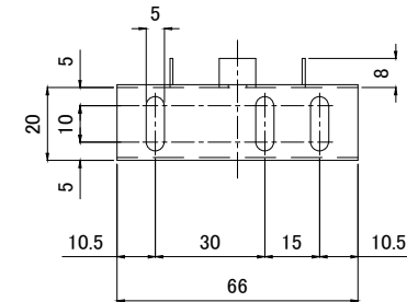
取付金具
