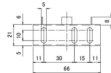
取付金具
